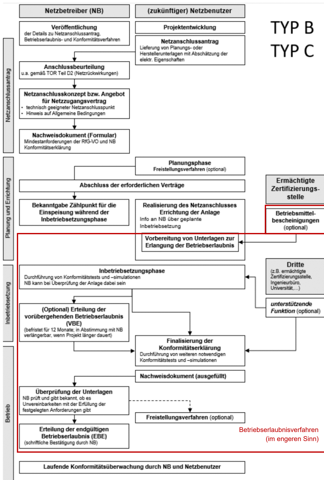
Abbildung 4: Grundsätzlicher Ablauf des Netzanschlussprozesses 1 insbesondere des Betriebserlaubnisverfahrens für Anlagen des Typs B und C 15
