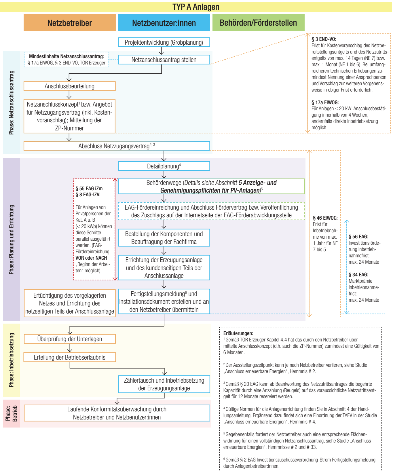
Abbildung 1: Schematischer Ablauf der Errichtung und des Betriebs von PV-Anlagen des Typs A in Anlehnung an TOR Erzeuger Typ A (Maximalkapazität <250 kW und Nennspannung <110 kV). Quelle: Photovoltaic Austria
