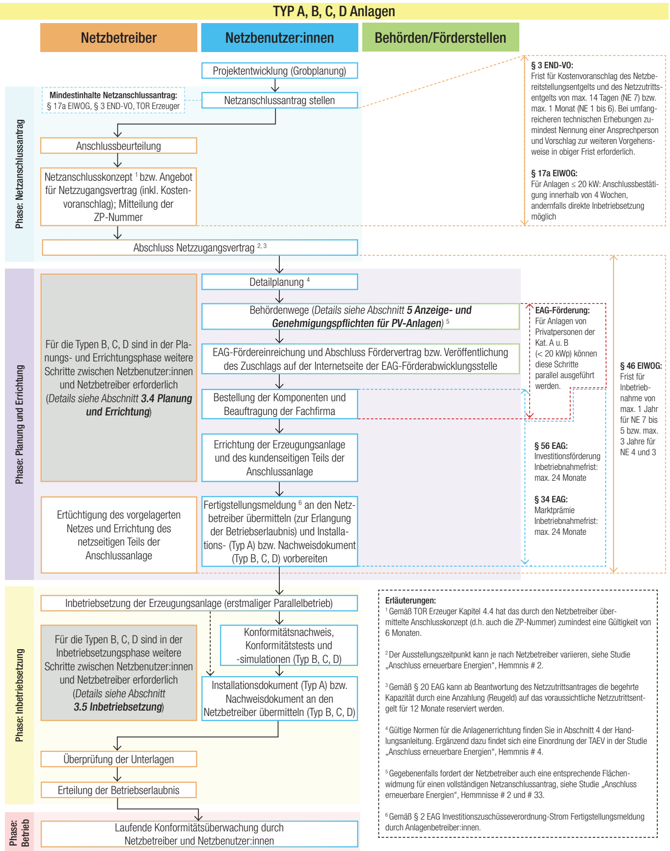
Abbildung 2: Schematischer Ablauf der Errichtung und des Betriebs von PV-Anlagen, in Anlehnung an TOR Erzeuger Anhang 4. Quelle: Photovoltaic Austria
