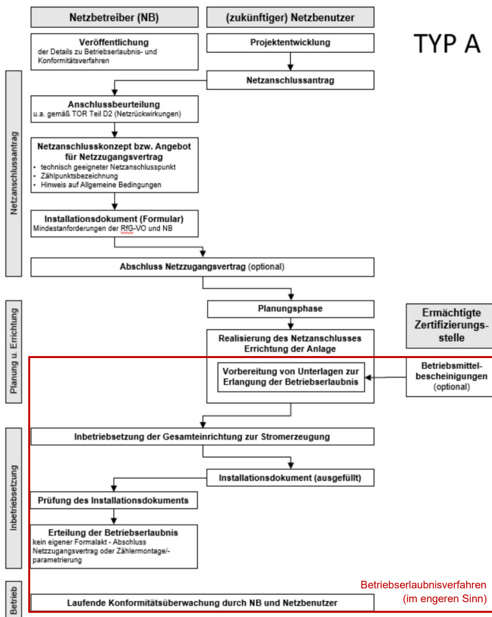
Abbildung 3: Grundsätzlicher Ablauf des Netzanschlussprozesses 1 insbesondere des Betriebserlaubnisverfahrens für Anlagen des Typs A und Kleinsterzeugungsanlagen 14
