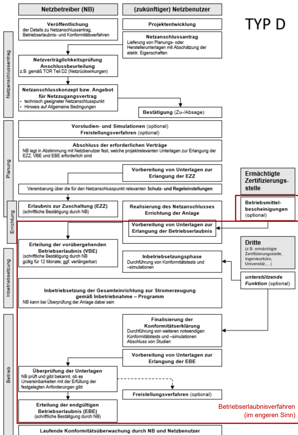
Abbildung 5: Grundsätzlicher Ablauf des Netzanschlussprozesses insbesondere des Betriebslaubnisverfahrens für Anlagen des Typs D 16
